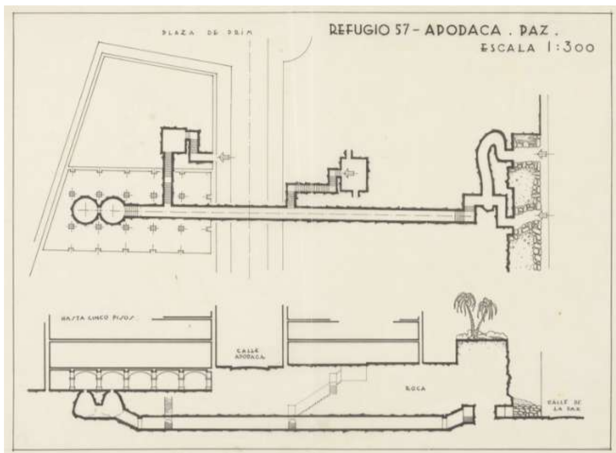
Imatge 98: Plànol del refugi 57 del carrer Apodaca de Tarragona. (Plànol extret de l'Arxiu Municipal de Tarragona)
