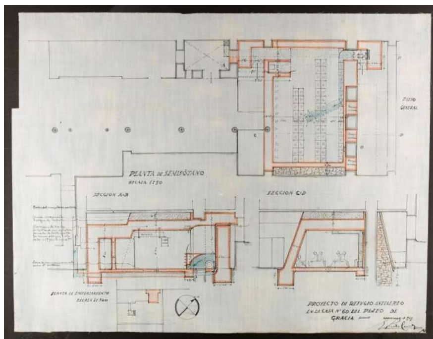
Imatge 5: Plànol del projecte tècnic per a la construcció d'un refugi antiaeri a l'edifici número 60 del passeig de Gràcia de Barcelona, seu del Govern d'Euskadi a Catalunya, redactat per l'arquitecte E. Pere Cendoya. (Imatge extreta de l'Arxiu Nacional de Catalunya)
