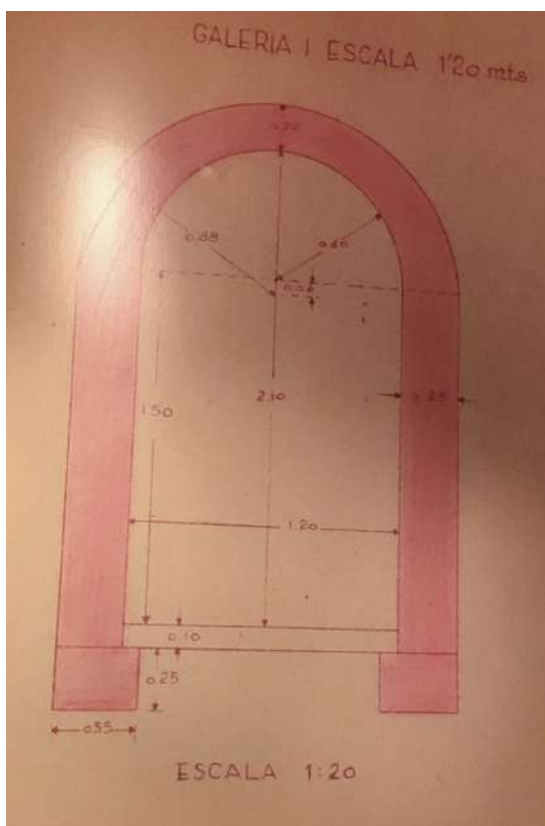
Imatge 36: Plànol de secció de la galeria del refugi de la patacada, on es veu la típica volta catalana. (Arxiu Municipal de Reus).
