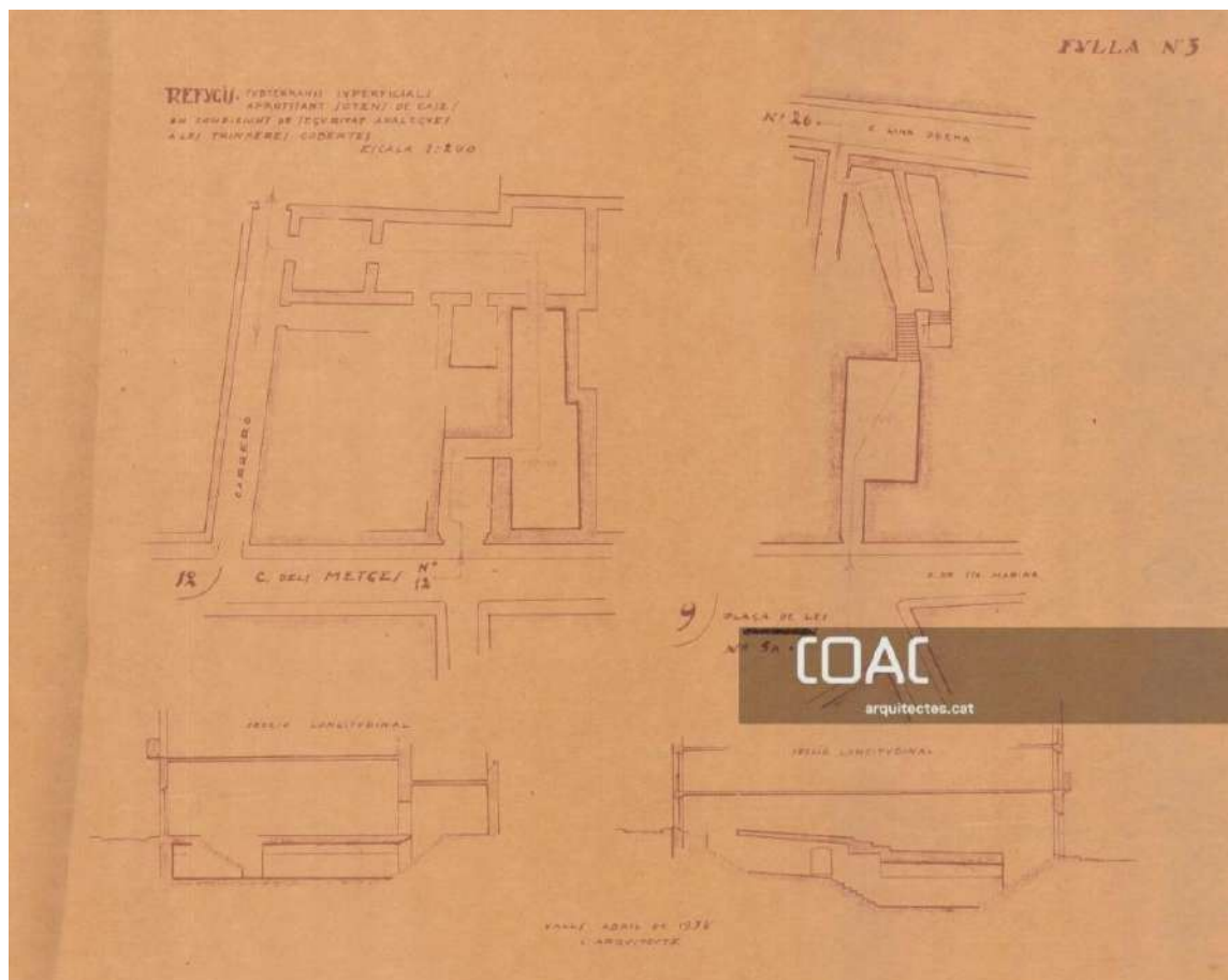
Imatge 11: Plànol d'un dels refugis antiaeris de Valls. (Col·legi d'Arquitectes de Catalunya).
