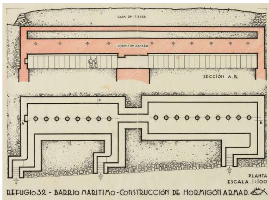
Imatge 50: Plànol del refugi 32 al Barri Marítim del Serrallo de Tarragona. (Arxiu Municipal de Tarragona).
