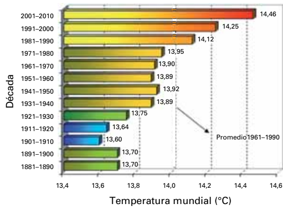
Figura 3. Promedio decenal mundial de la temperatura tierra-océano en superficie (°C) basado en tres conjuntos de valores de la temperatura mundial (Fuente: Centro Hadley de la Oficina Meteorológica de Reino Unido y Unidad de Investigación sobre el Clima de la Universidad de East Anglia, Reino Unido)
