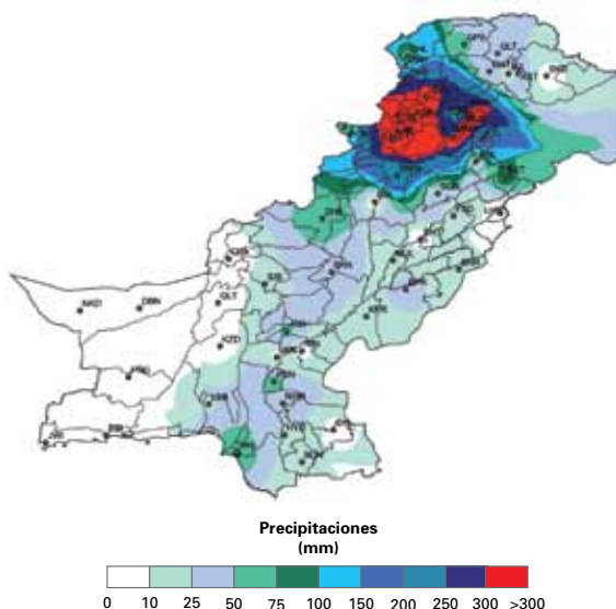
Figura 9. Precipitaciones (mm) en Pakistán entre el 26 y 29 de julio de 2010 (Fuente: Departamento de Meteorología de Pakistán)
