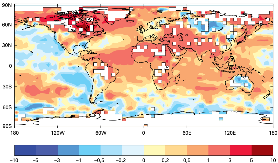
Figura 4. Anomalías de la temperatura mundial en la superficie del mar y de la tierra (°C) en 2010 respecto del período de 1961-1990 (Fuente: Centro Hadley de la Oficina Meteorológica de Reino Unido y Unidad de Investigación sobre el Clima de la Universidad de East Anglia, Reino Unido)
